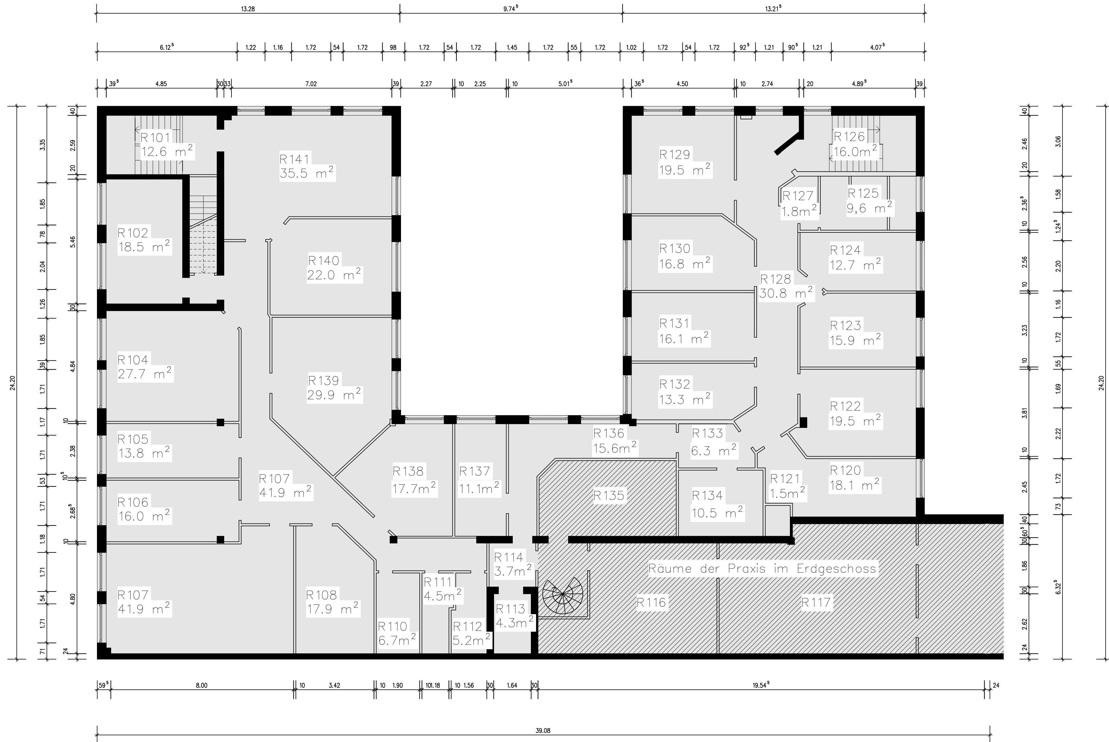
1. Obergeschoss
